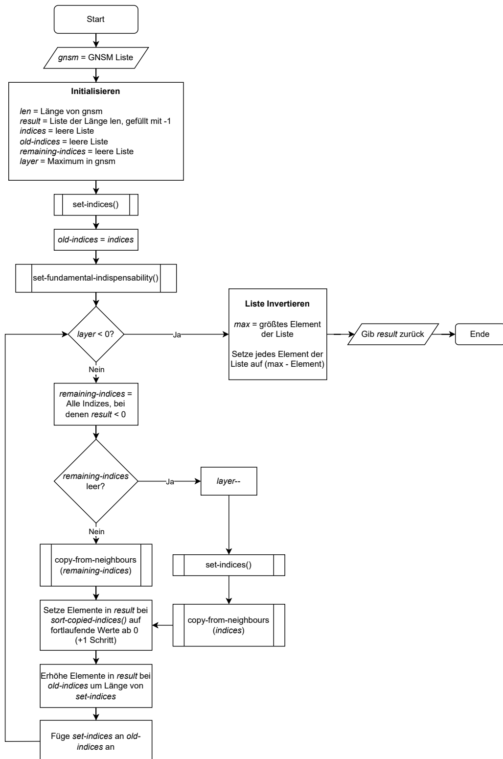
Abbildung 3.7.: Programmablaufplan für die Funktion gns-to-indispensability-list .
