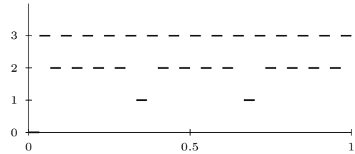
(b) Die get-metrical-depth Funktion für ein Metrum definiert durch (3 5 2), also 3x5x2.
